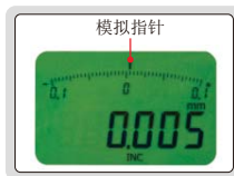
模拟指针显示
