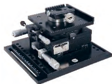
轮廓仪夹具
